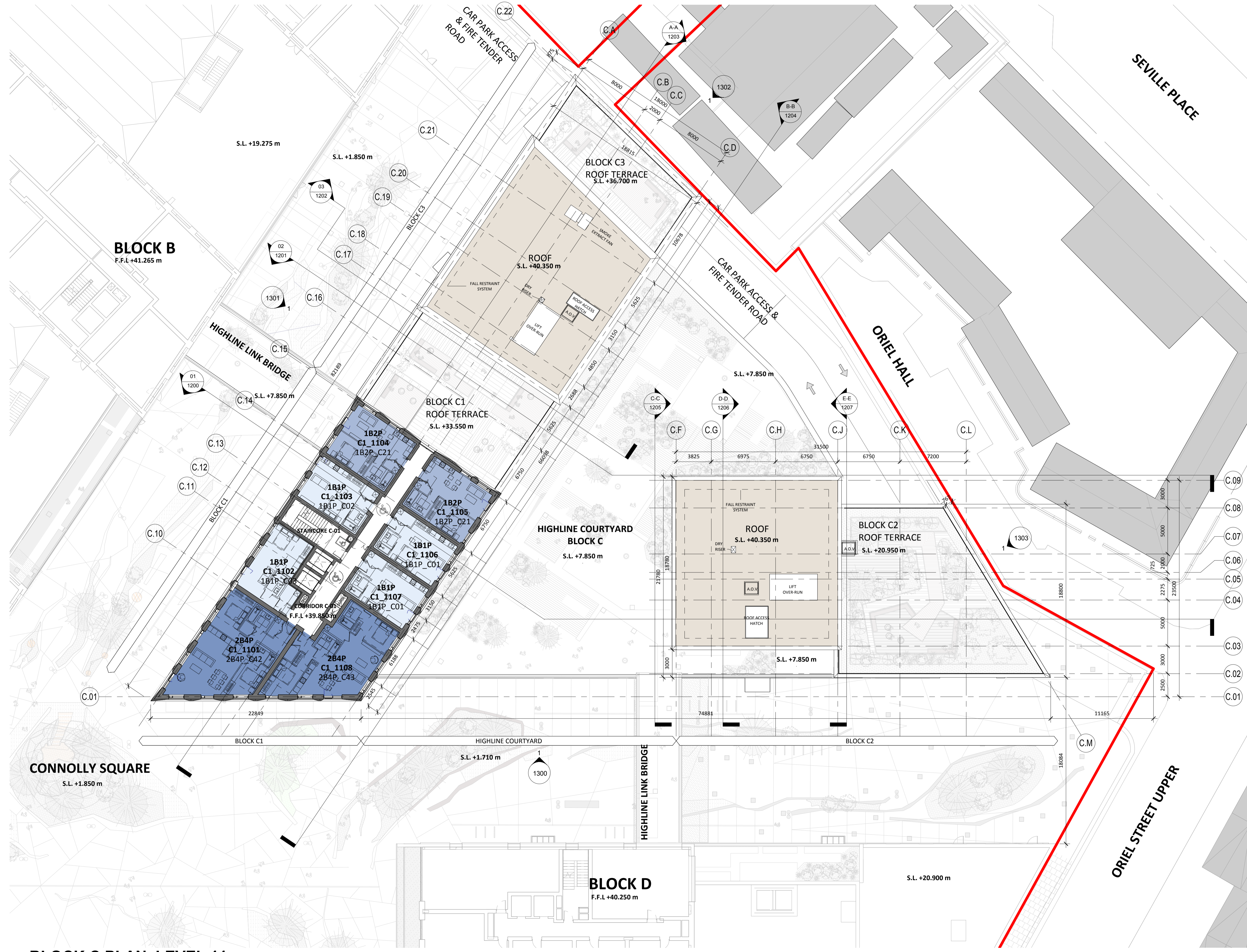
1 BLOCK C PLAN_LEVEL 11 1 : 200
